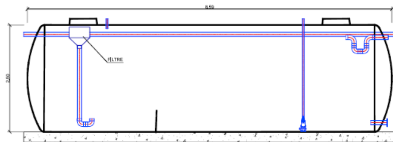
DETTALL DEPÒSIT E.180
