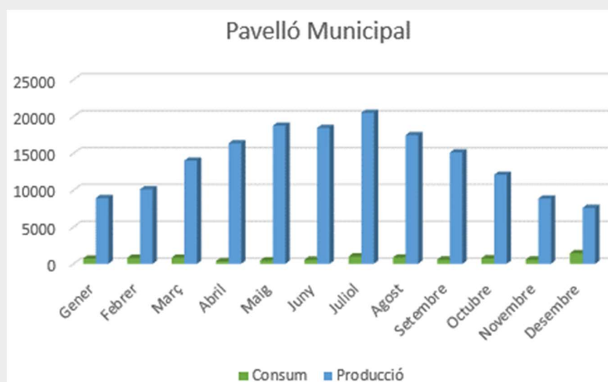
Figura 9. Representació gràfica consum vs. producció del Pavelló municipal Font: Elaboració pròpia
