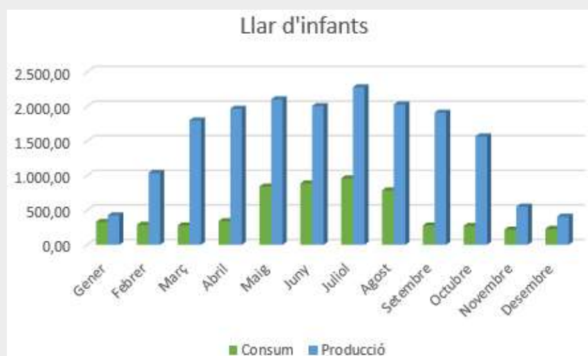
Figura 15. Representació gràfica consum vs. producció de la Llar d'infants Font: Elaboració pròpia
