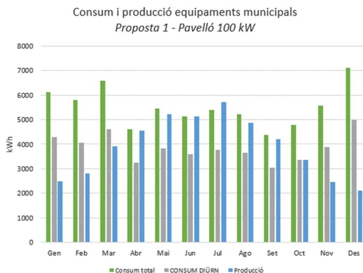
Figura 33. Gràfic consum i producció equipaments municipals
