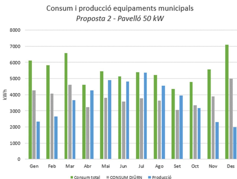
Figura 36. Gràfic consum i producció equipaments municipals
