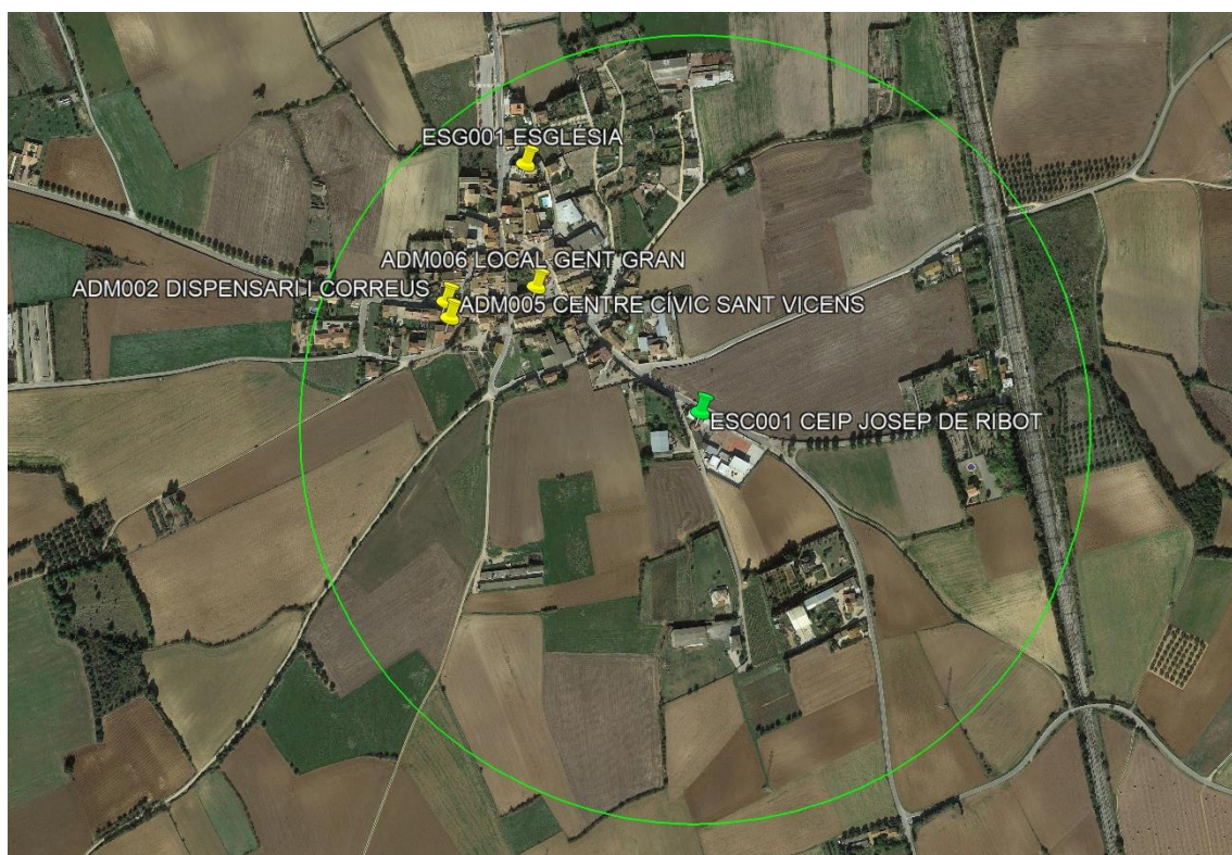
Figura 13. Equipaments associats i radi d'actuació Instal·lació FV 3 amb el sistema d'emmagatzematge. Font: elaboració pròpia i Google Earth.
