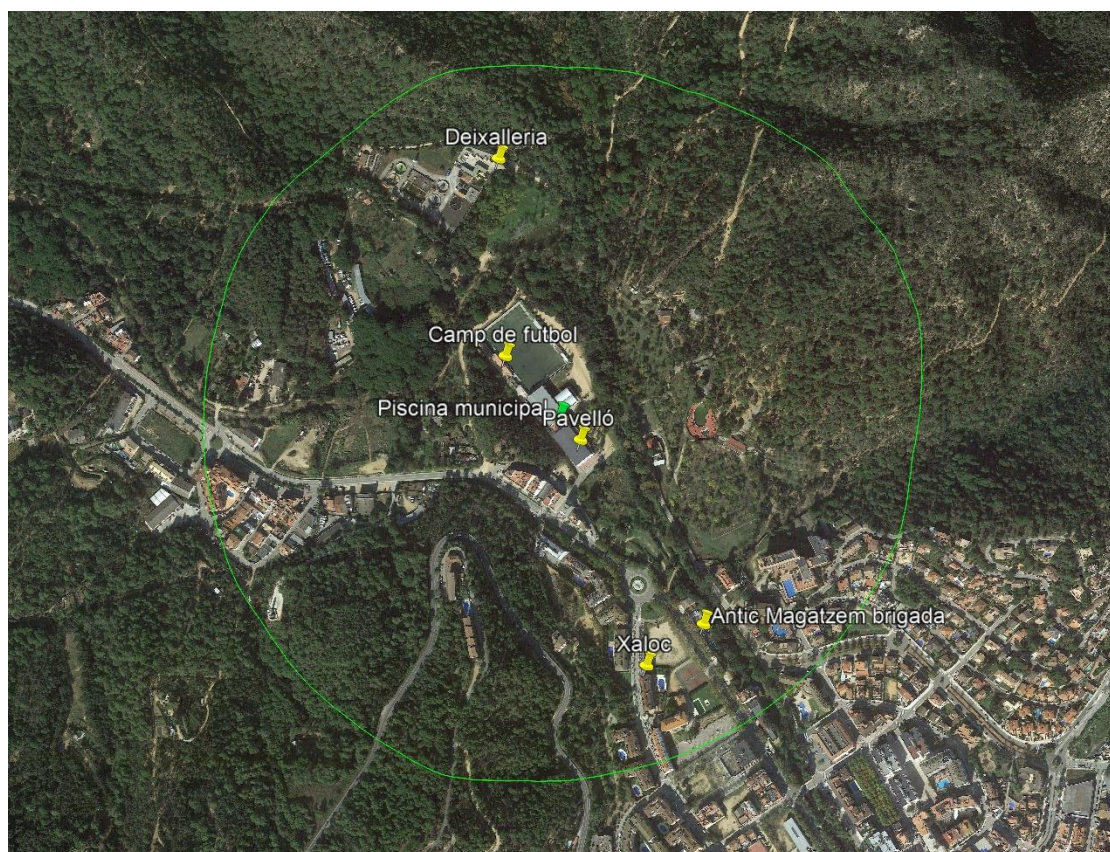
Figura 11. Equipaments associats i radi d'actuació Instal·lació FV 3 amb el sistema d'emmagatzematge. Font: elaboració pròpia i Google Earth.
