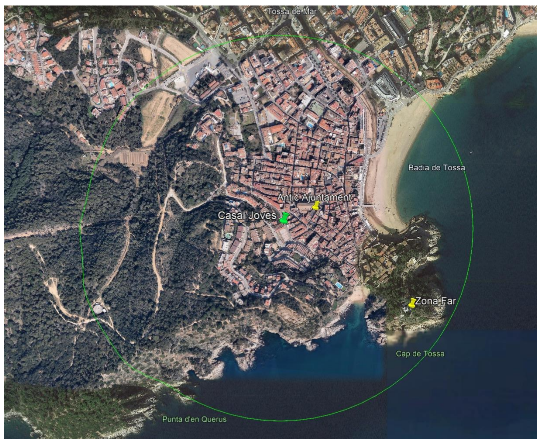
Figura 8. Equipaments associats i radi d'actuació Instal·lació FV 2. Font: elaboració pròpia i Google Earth.
