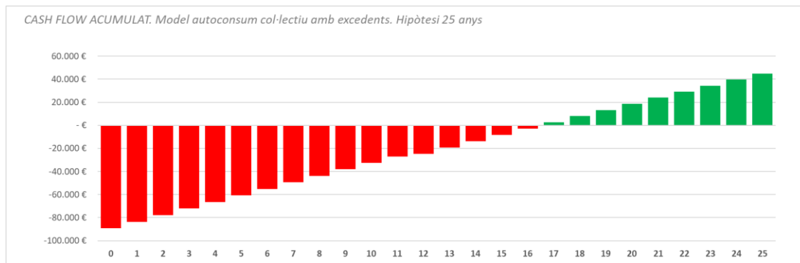
Figura 8. Gràfic del cash-flow durant els primers 25 anys de la instal·lació FV proposada. Font: Elaboració pròpia.
