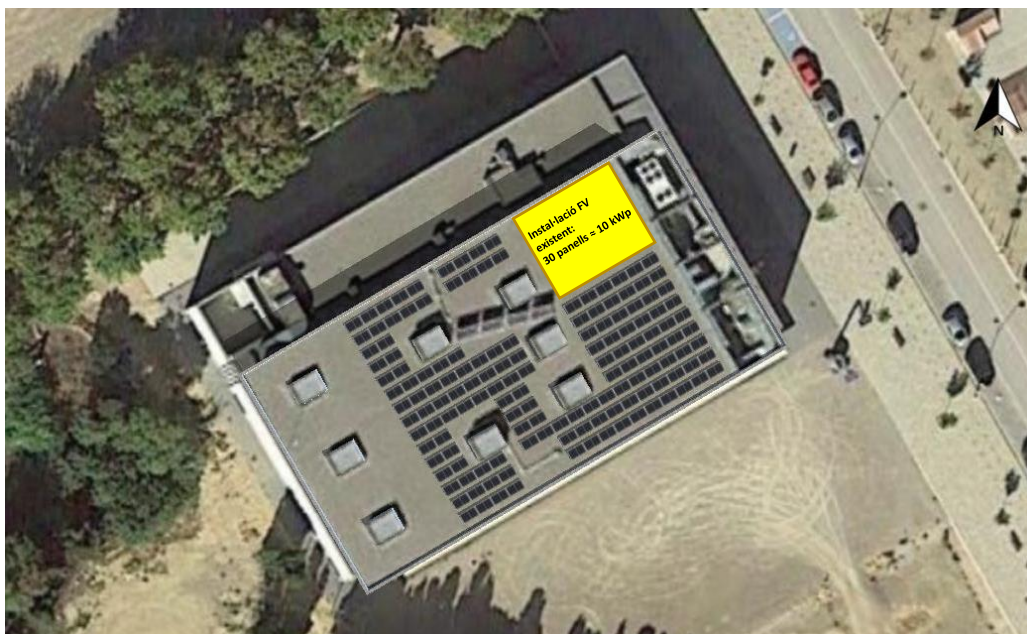
Figura 7. Imatge en 3D de la instal·lació FV plantejada 2. Font: PVSOL.
