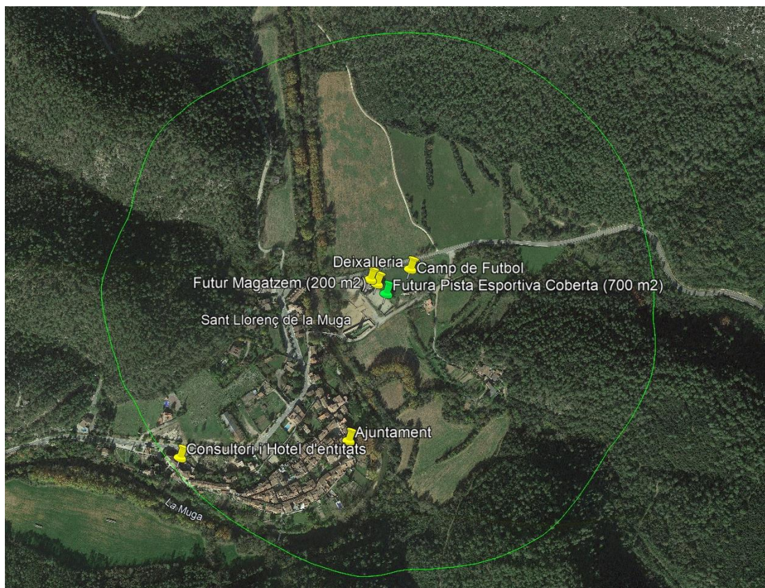
Figura 9. Equipaments associats i radi d'actuació Instal·lació FV 1 amb el sistema d'emmagatzematge. Font: elaboració pròpia i Google Earth.
