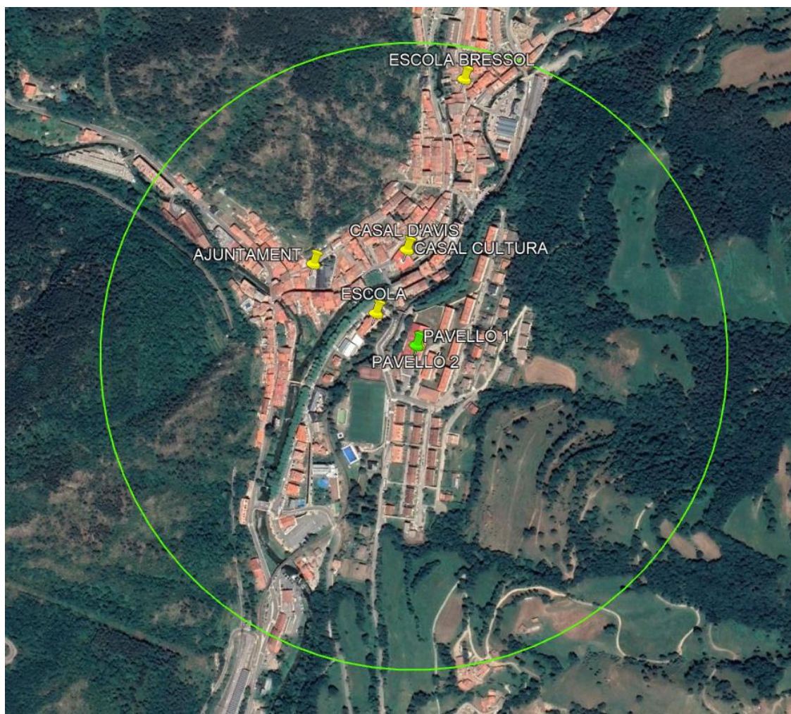
Figura 6. Equipaments associats i radi d'actuació Instal·lació FV 1. Font: elaboració pròpia i Google Earth.
