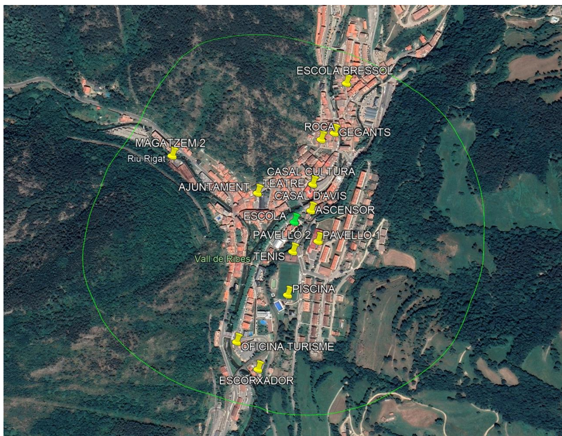
Figura 10. Equipaments associats i radi d'actuació Instal·lació FV 3. Font: elaboració pròpia i Google Earth.
