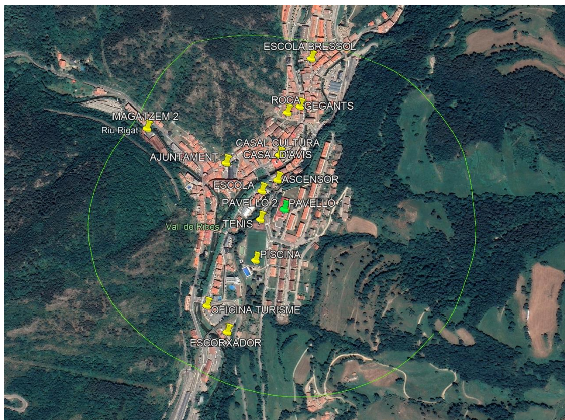
Figura 8. Equipaments associats i radi d'actuació Instal·lació FV 2. Font: elaboració pròpia i Google Earth.
