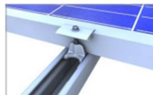
Pinza intermedia en el rail C47
