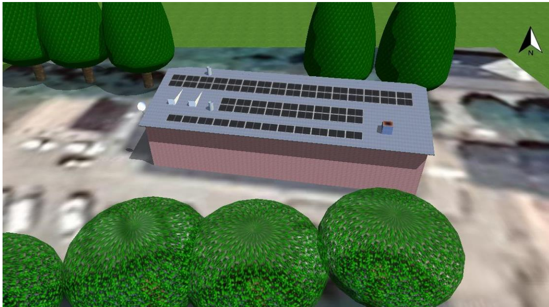
Figura 5. Imatge en 3D de la instal·lació FV plantejada 1. Font: PVSOL.
