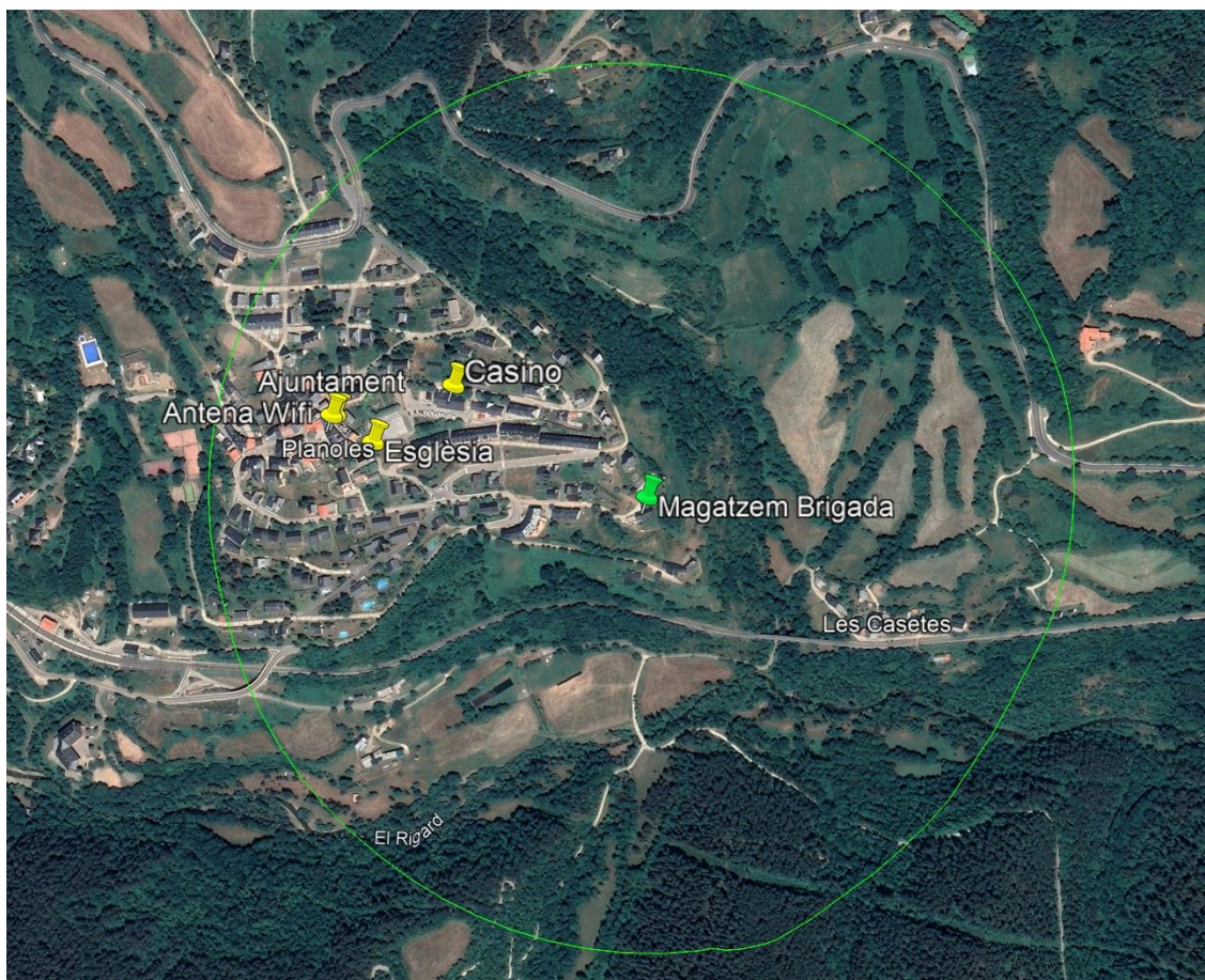
Figura 9. Equipaments associats i radi d'actuació Instal·lació FV 2. Font: elaboració pròpia i Google Earth.
