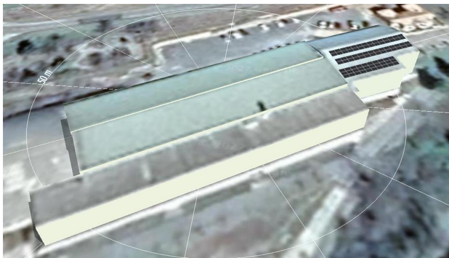
Figura 4. Imatge en 3D de la instal·lació FV plantejada 1. Font: PVSOL.
