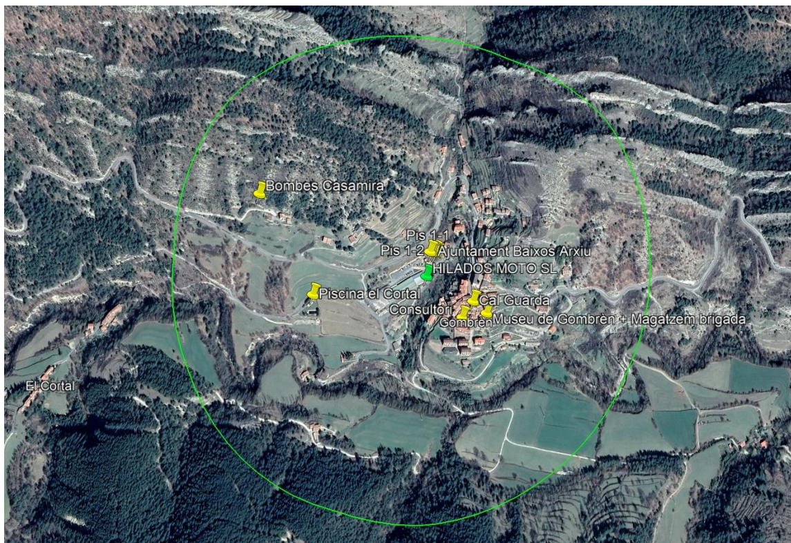
Figura 9. Equipaments associats i radi d'actuació Instal·lació FV 1+2 amb el sistema d'emmagatzematge. Font: elaboració pròpia i Google Earth.
