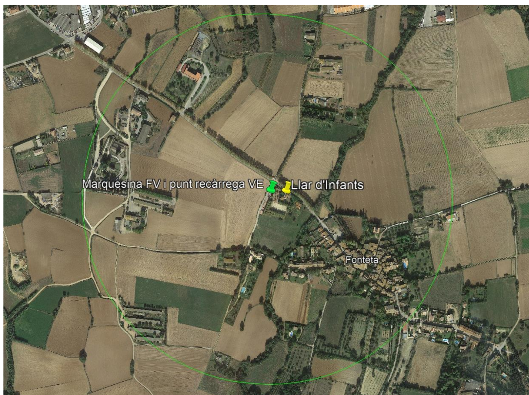
Figura 9. Equipaments associats i radi d'actuació Instal·lació FV 2 amb el punt de recàrrega de VE. Font: elaboració pròpia i Google Earth.
