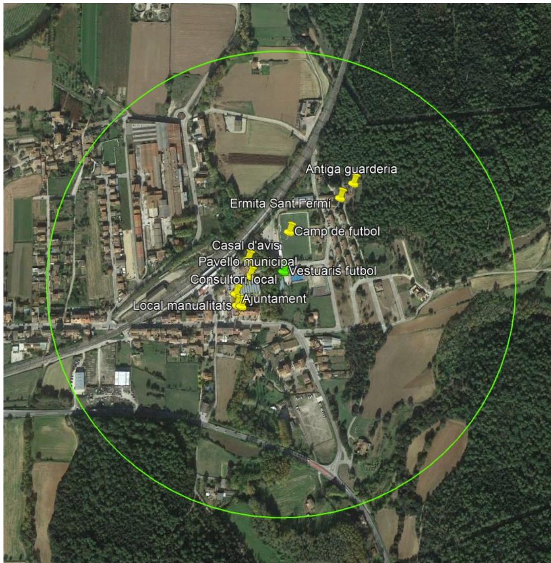
Figura 9. Equipaments associats i radi d'actuació Instal·lació FV 2. Font: elaboració pròpia i Google Earth.
