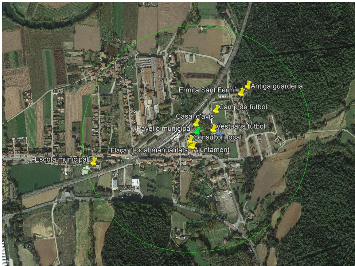
Figura 7. Equipaments associats i radi d'actuació Instal·lació FV 1. Font: elaboració pròpia i Google Earth.
