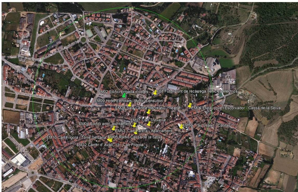
Figura 10. Equipaments associats i radi d'actuació Instal·lació FV 2 amb el sistema d'emmagatzematge. Font: elaboració pròpia i Google Earth.
