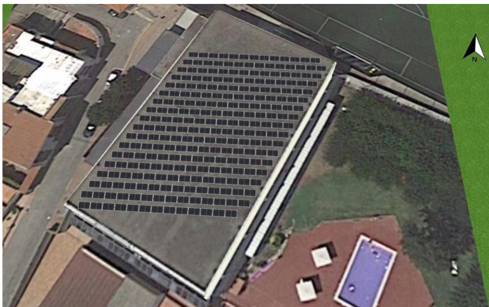
Figura 4. Imatge en 3D de la instal·lació FV plantejada 1. Font: PVSOL.
