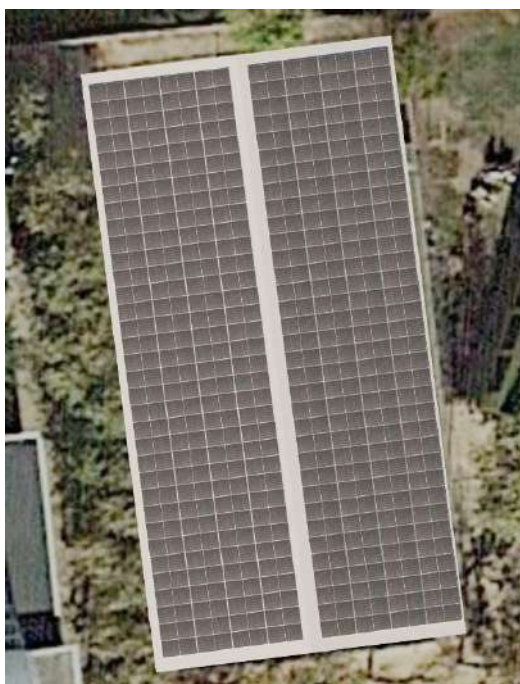
Imatge 17. Proposta d'instal·lació si es cobreix la pista de l'Escola Llagut.
