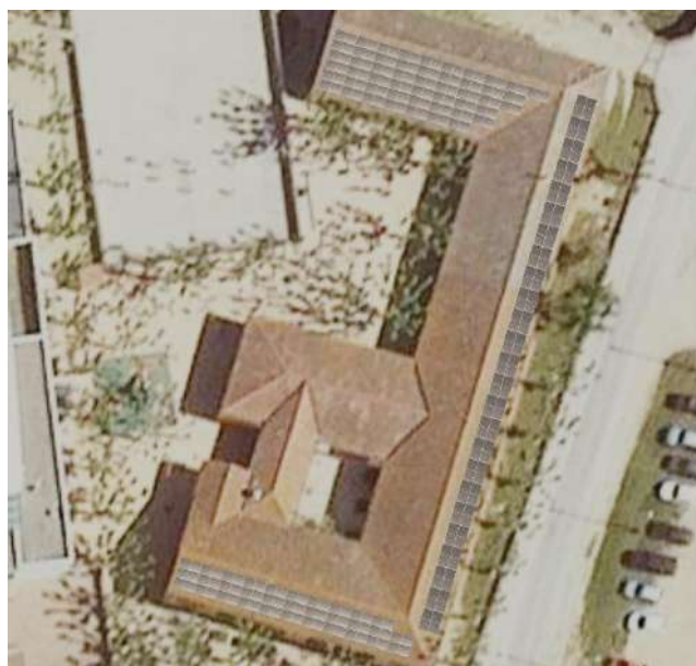
Imatge 15. Proposta d'instal·lació a la coberta de l'Escola Llagut.
