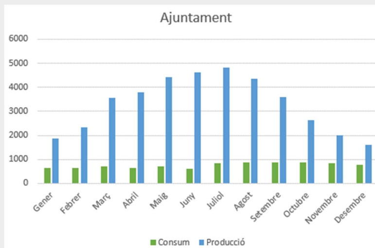
Figura 8. Representació gràfica consum vs. producció Ajuntament Font: Elaboració pròpia
