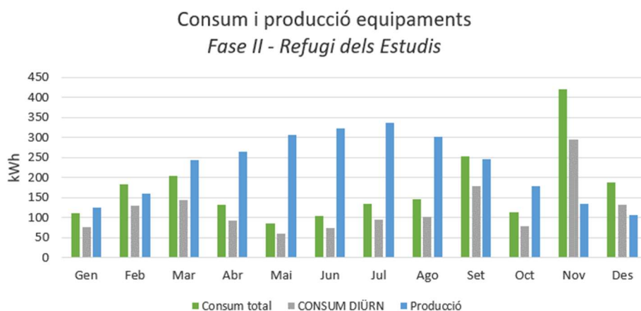
Figura 28. Gràfic consum i producció equipaments municipals Fase II Font: Elaboració pròpia
