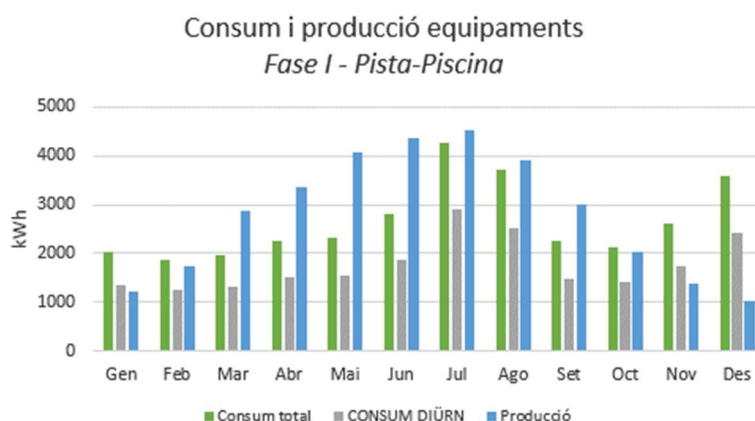
Figura 20. Gràfic consum i producció equipaments municipals Fase I
