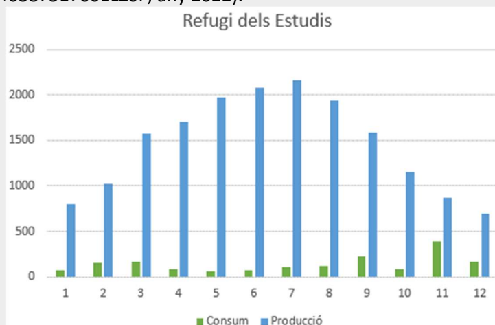
Figura 11. Representació gràfica consum vs. producció Refugi dels Estudis Font: Elaboració pròpia
