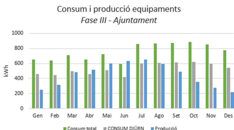
Figura 31. Gràfic consum i producció equipaments municipals Fase III
