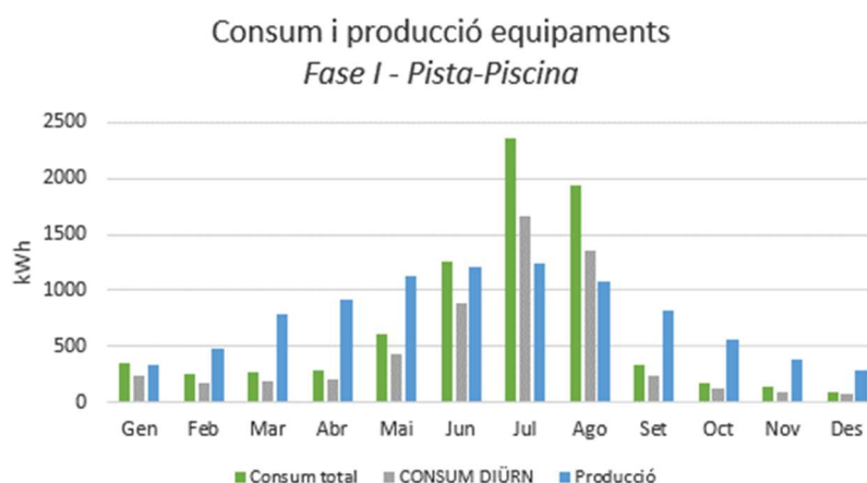
Figura 25. Gràfic consum i producció equipaments municipals Fase I
