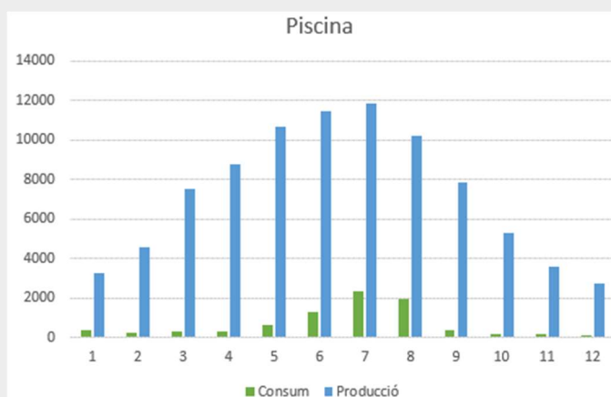
Figura 14. Representació gràfica consum vs. producció Pista-Piscina Font: Elaboració pròpia
