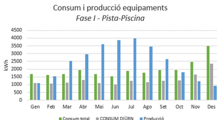
Figura 22. Gràfic consum i producció equipaments municipals Fase I
