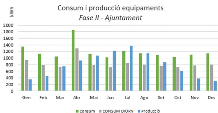
Figura 28. Gràfic consum i producció equipaments municipals
