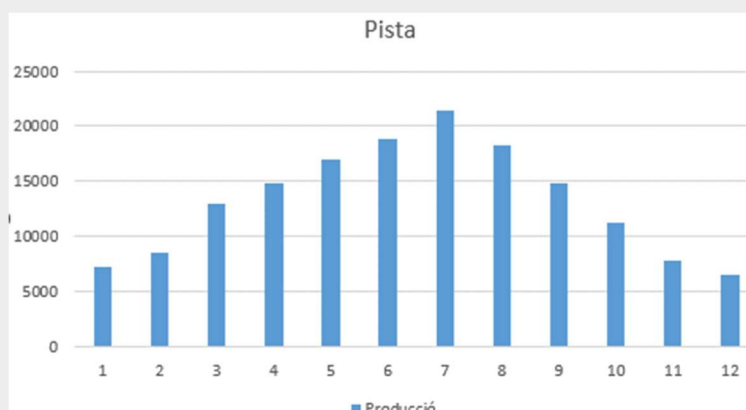
Figura 17. Representació gràfica consum vs. producció de Pista Font: Elaboració pròpia
