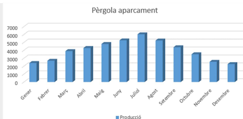
Figura 20. Representació gràfica producció de la Pèrgola aparcament Font: Elaboració pròpia
