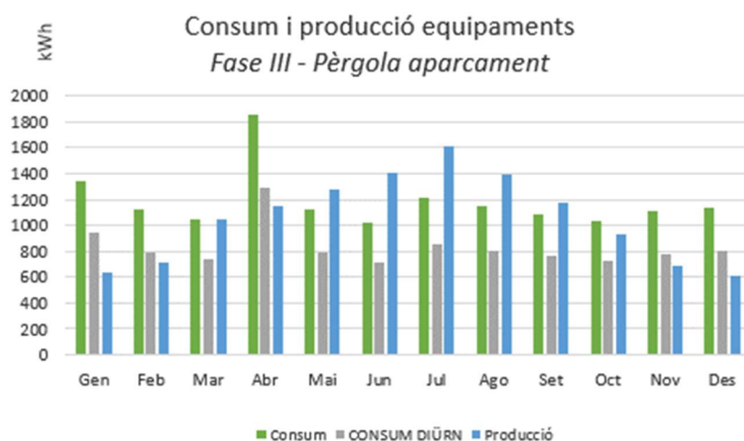
Figura 31. Gràfic consum i producció equipaments municipals
