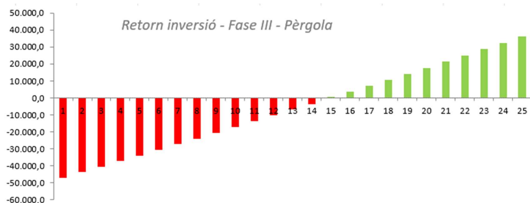
Figura 30. Gràfic del retorn de la inversió
