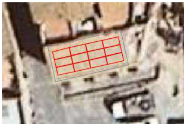
Imatge 16. Proposta d'instal·lació de panells a la coberta de l'Ajuntament.
