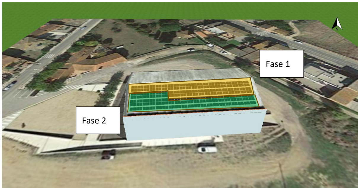
Figura 6. Imatges en 3D de les instal·lacions FV 2 plantejades. Font: PVSOL.
