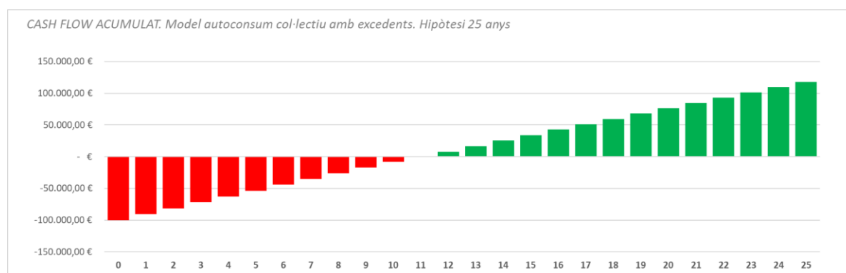
Figura 15. Gràfic del cash-flow durant els primers 25 anys de la instal·lació FV. Font: Elaboració pròpia.
