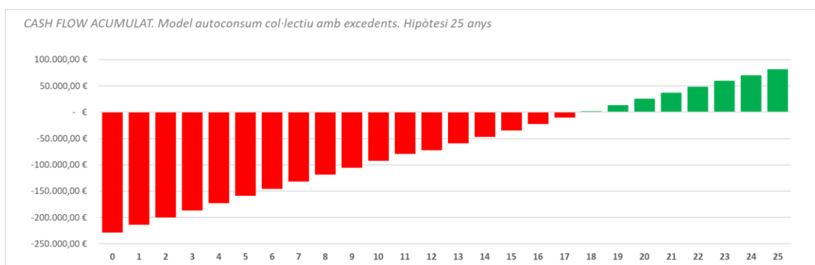
Figura 17. Gràfic del cash-flow durant els primers 25 anys de la instal·lació FV. Font: Elaboració pròpia.
