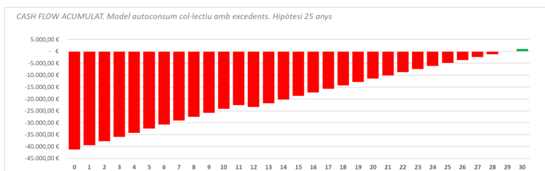
Figura 12. Gràfic del cash-flow durant els primers 25 anys de la instal·lació FV 1. Font: Elaboració pròpia.
