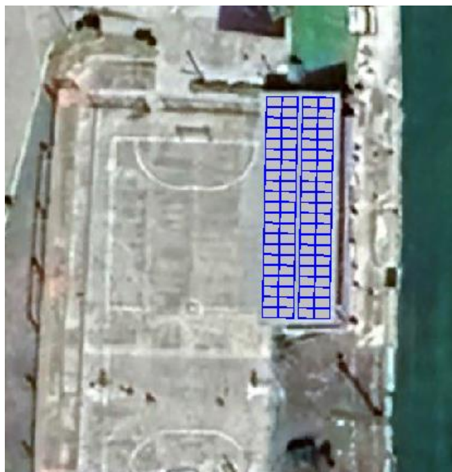
Figura 6. Croquis de la instal·lació fotovoltaica.
