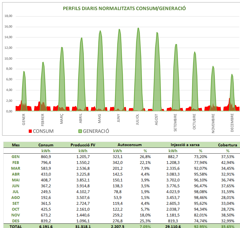
Figura 9. Consum i generació Escola.
