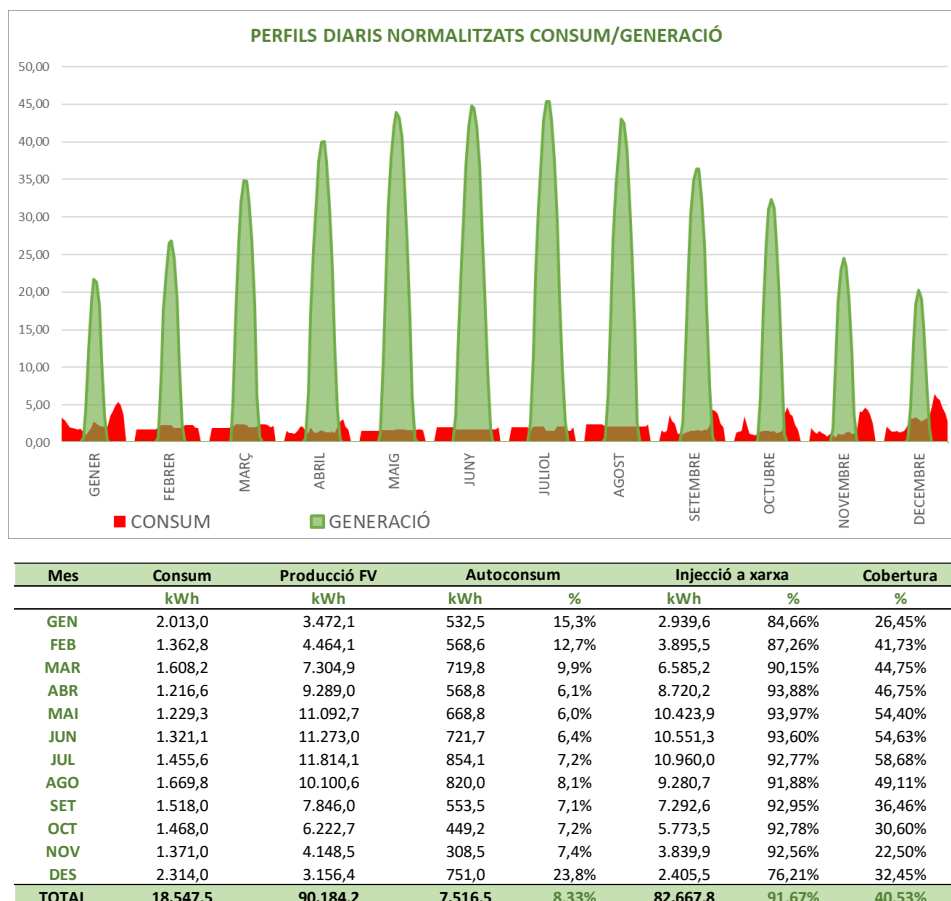
Figura 5. Consum i generació Zona Esportiva (Sala i Bar).
