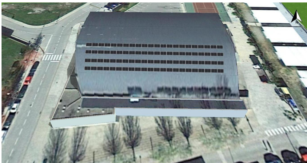
Figura 4. Imatge en 3D de la instal·lació FV plantejada 1. Font: PVSOL.
