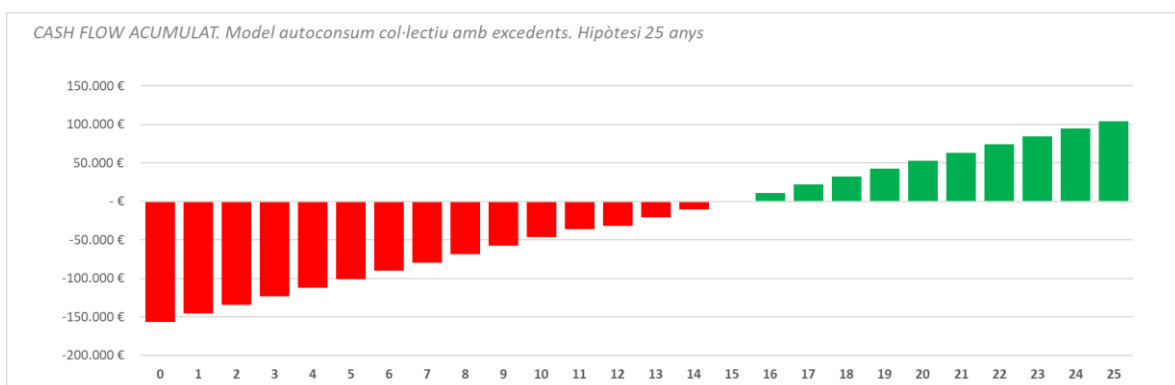
Figura 7. Gràfic del cash-flow durant els primers 25 anys de la instal·lació FV proposada. Font: Elaboració pròpia.
